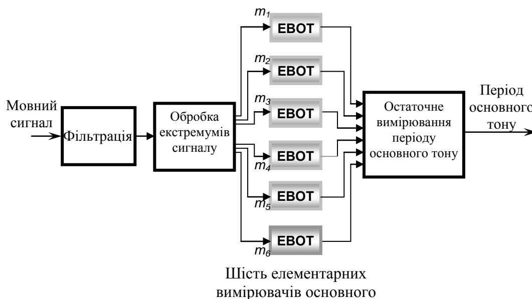
Рис. 1. Блок-схема визначника основного тону
